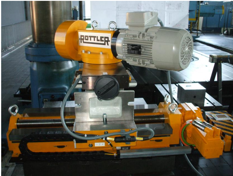
Lösung: Transportable Bearbeitungseinheit TB, hier mit aufgebauter Schleifeinheit
